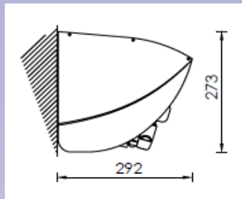
Montage façade avec auvent
