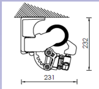
Montage pose plafond
