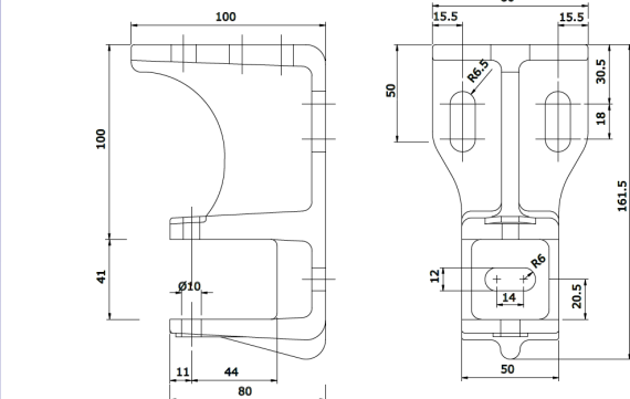
BRIDE MUR / PLAFOND EN FONTE
