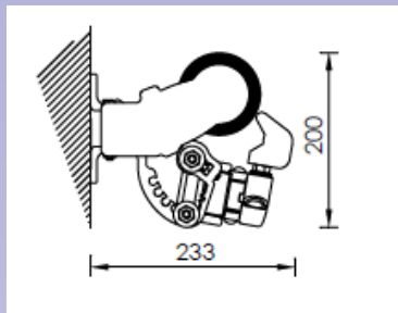
Montage pose façade
